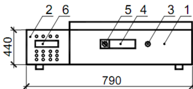
Рисунок 1.1 - Схема лабораторной установки: 1 – пылевая камера; 2 – приборный отсек; 3 – отверстие для взятия пробы; 4 – прозрачное окно; 5 – ручка дозатора; 6 – аспиратор А-822.
