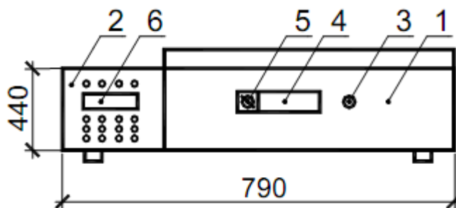
Рисунок 1.1 - Схема лабораторной установки: 1 – пылевая камера; 2 – приборный отсек; 3 – отверстие для взятия пробы; 4 – прозрачное окно; 5 – ручка дозатора; 6 – аспиратор А-822.
