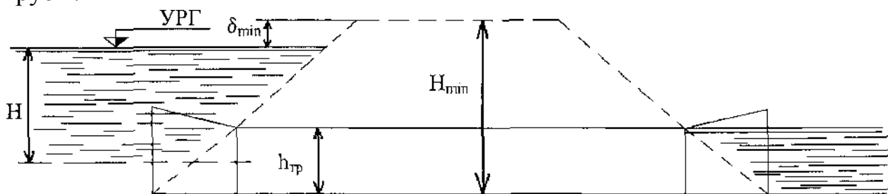
Рис. 1 Схема трубы.
