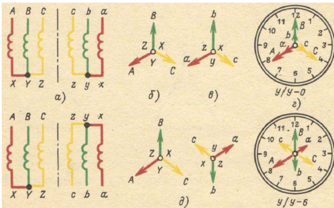
Рисунок 9. Примеры определения группы соединения при включении обеих обмоток в звезду.
