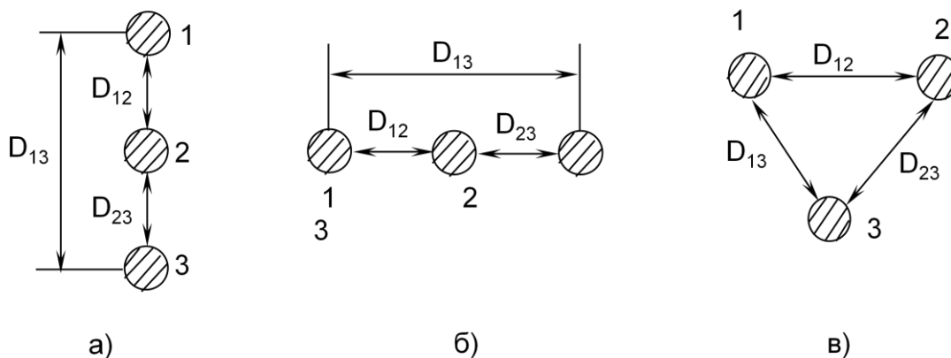
Рисунок 4.3 – Расположение проводов на опоре:
