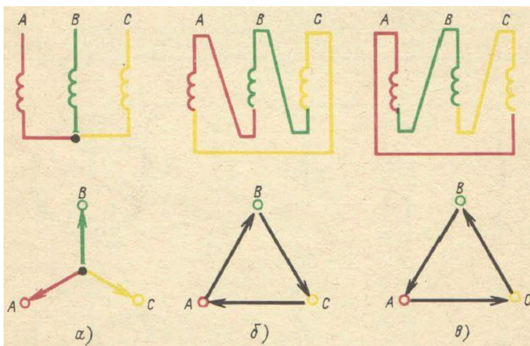
Рисунок 11. Расположение векторов при соединении в треугольник обмоток ВН.
