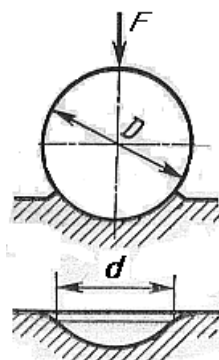
Рис. 1 – Схема определения твердости по методу Бринелля
