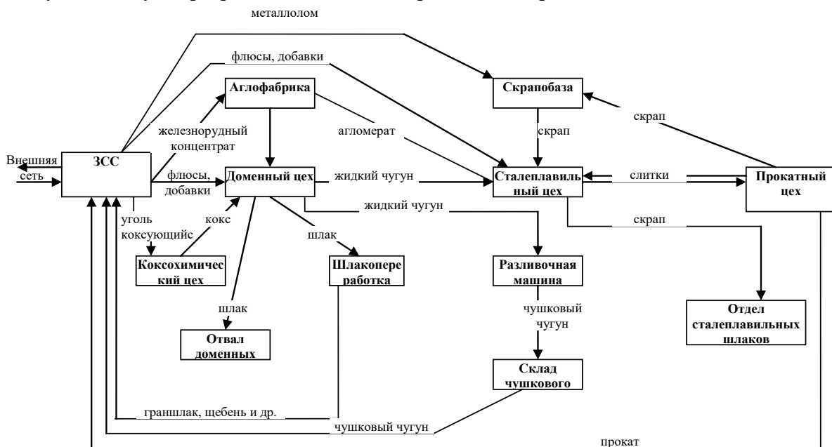
Рисунок 1.1 – Схема технологических взаимосвязей металлургического завода
