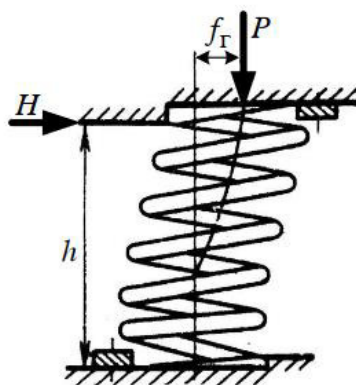
Рисунок 1 – Положение пружины при действии вертикальной и горизонтальной нагрузок
