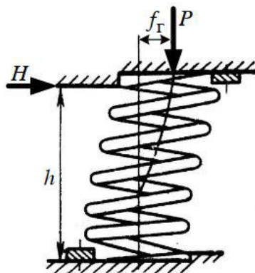
Рисунок 1 – Положение пружины при действии вертикальной и горизонтальной нагрузок
