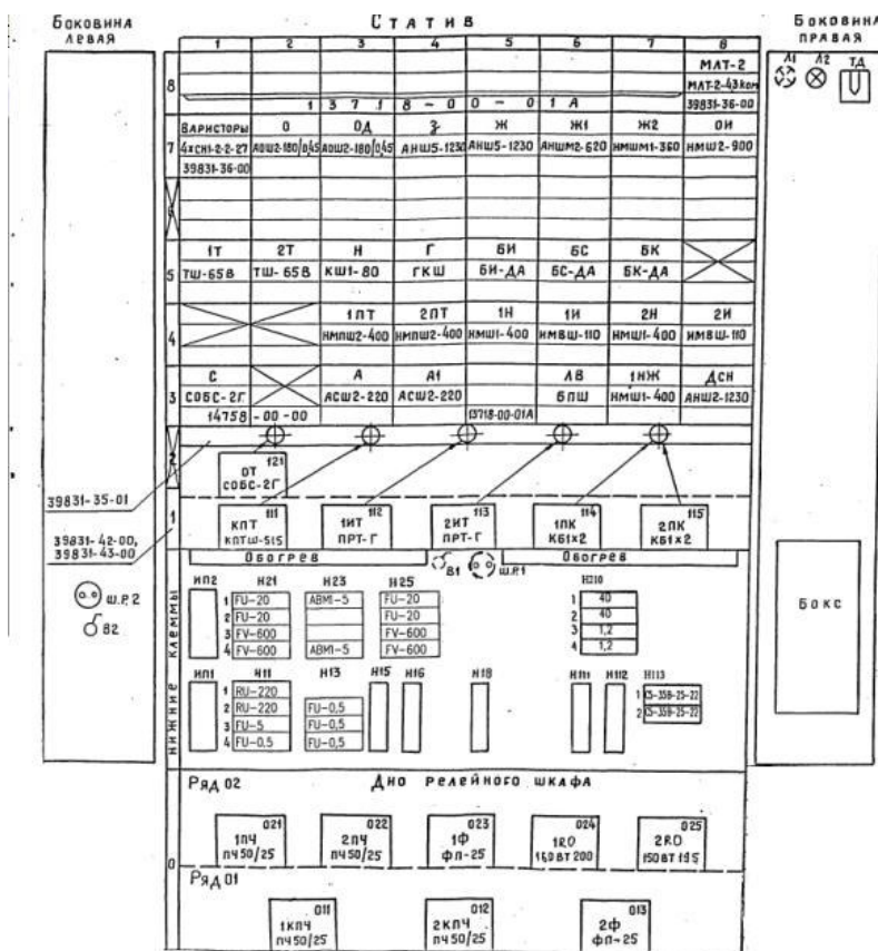
Рис.П1. Комплектование и монтаж шкафа релейного унифицированного ШРУ-М (410115-ГМП «Комплектование и монтаж шкафов релейных унифицированных типа ШРУ-М»)
