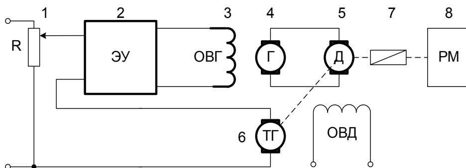
Рис.1. Принципиальная схема САУ
