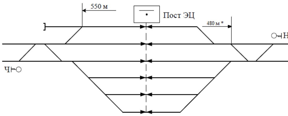
Рисунок 1 – Схема станции
