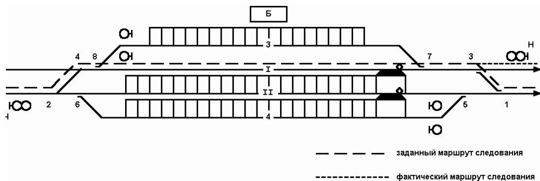
Рис. 4.5. Положение на путях станции
