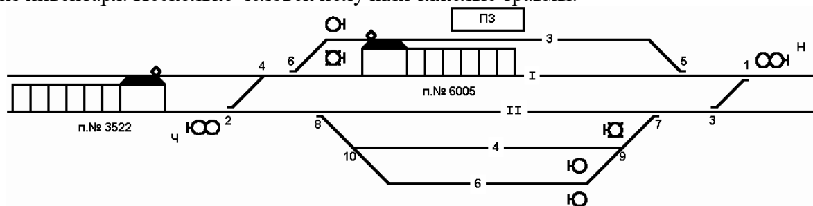
Рис. 4.1. Расположение поездов перед столкновением
