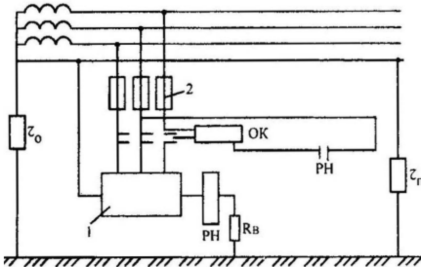
Рис. 2. Схема устройства защитного отключения: 1 – корпус электроустановки; 2 – предохранители; ОК – отключающая катушка автоматического выключателя; РН – реле напряжения; z_0 – сопротивление заземления нейтрали; R_B – сопротивление вспомогательного заземления; z_n – сопротивление повторного заземления
