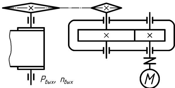
Рисунок 1 – Схема привода
