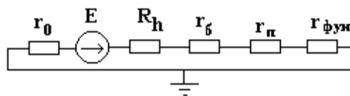
Эквивалентная схема
