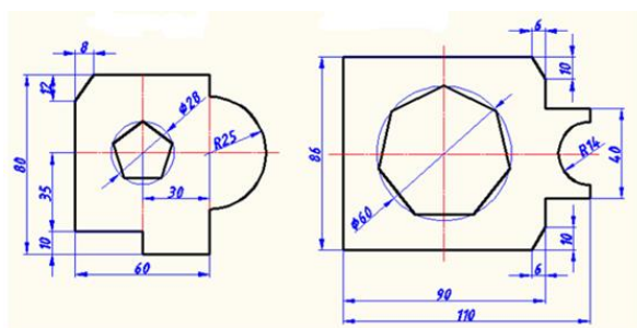
Проекционный чертеж детали
