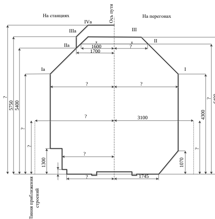
Габарит приближения строений
