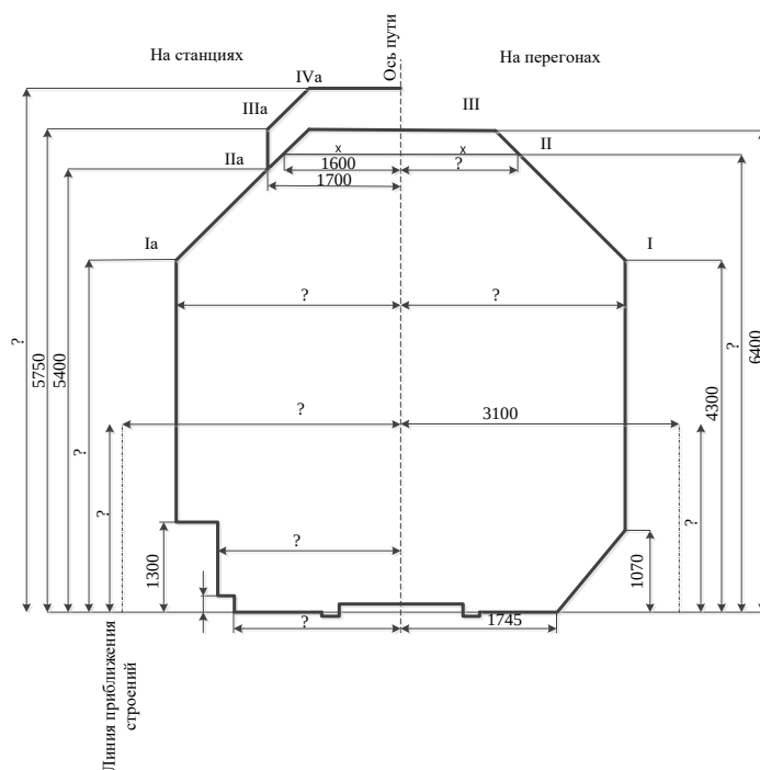
Габарит приближения строений
