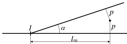
Рис. 1 - Основная схема установки предельного столбика
