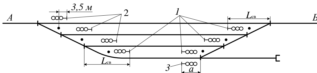
Рис. 4 - Случаи установки выходных светофоров
