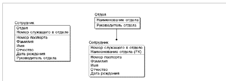
Рисунок 5 - Иллюстрация второй нормальной формы
