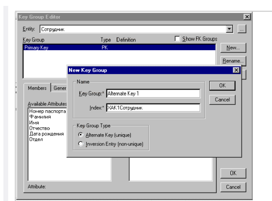
Рисунок 3 - Диалог Key Group Editor
