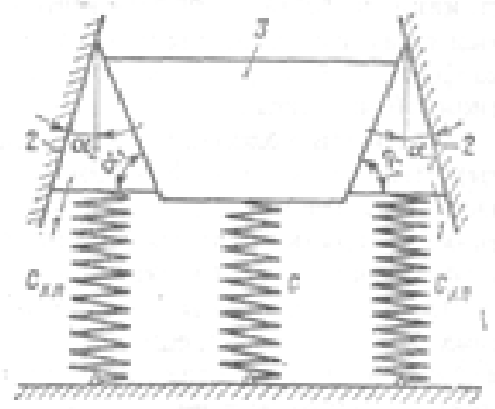
Рис. 1 Схема клинового гасителя колебаний
