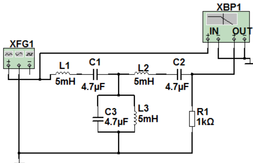
Рис. 11.9. Фильтр полосовой
