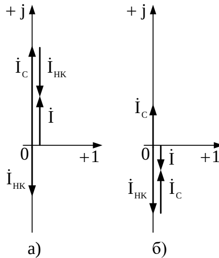
Рис. 18.2. Векторные диаграммы токов: I_C > I_{HK} (а) и I_C < I_{HK} (б)
