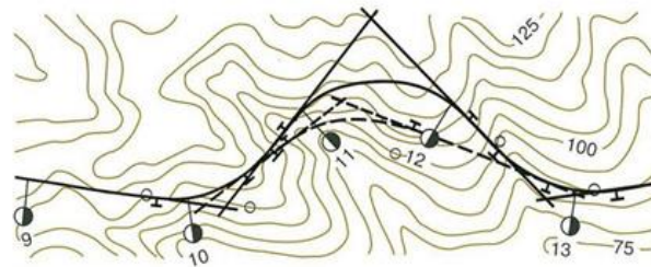
План трассы
