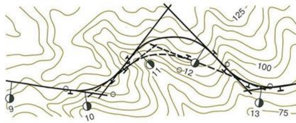
План трассы
