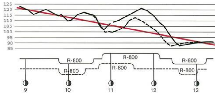
Продольный профиль
