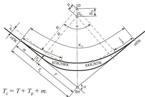
Элементы круговой и переходных кривых
