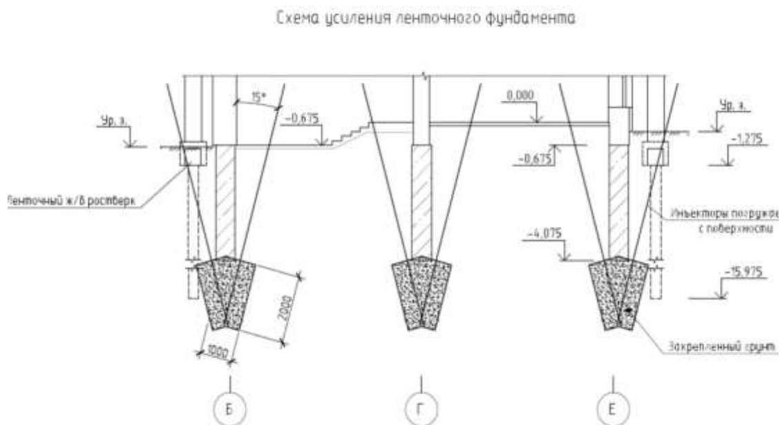
Рисунок 1 – Схема усиления ленточного фундамента свайными фундаментами
