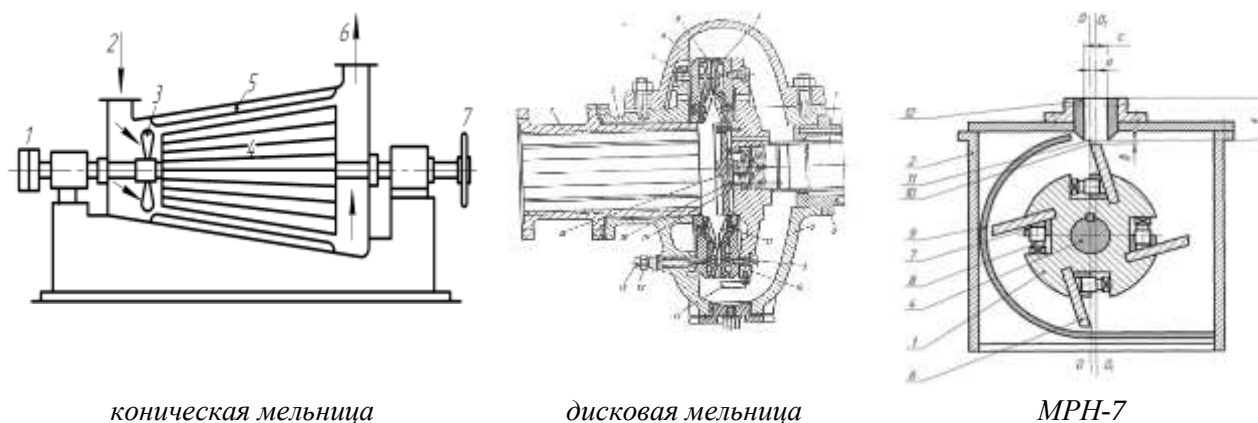
Рисунок 1 – Лабораторные размольные установки
