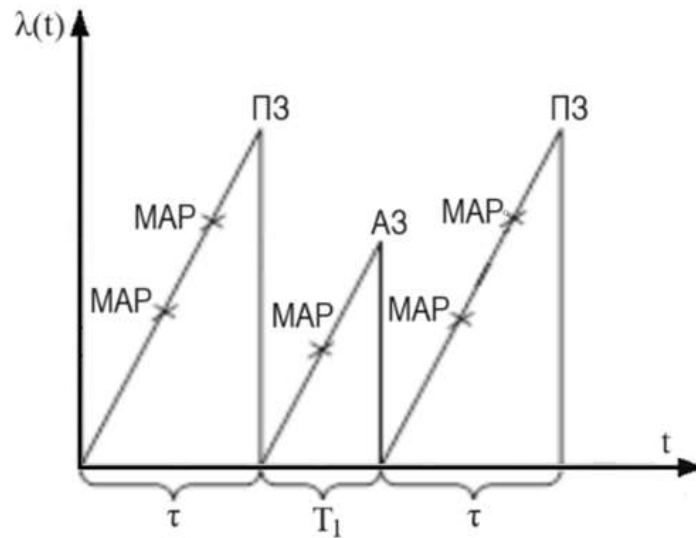
Рисунок 2 – Зависимость интенсивности отказов \lambda(t) от проведения во время эксплуатации МАР, АЗ и ПЗ
