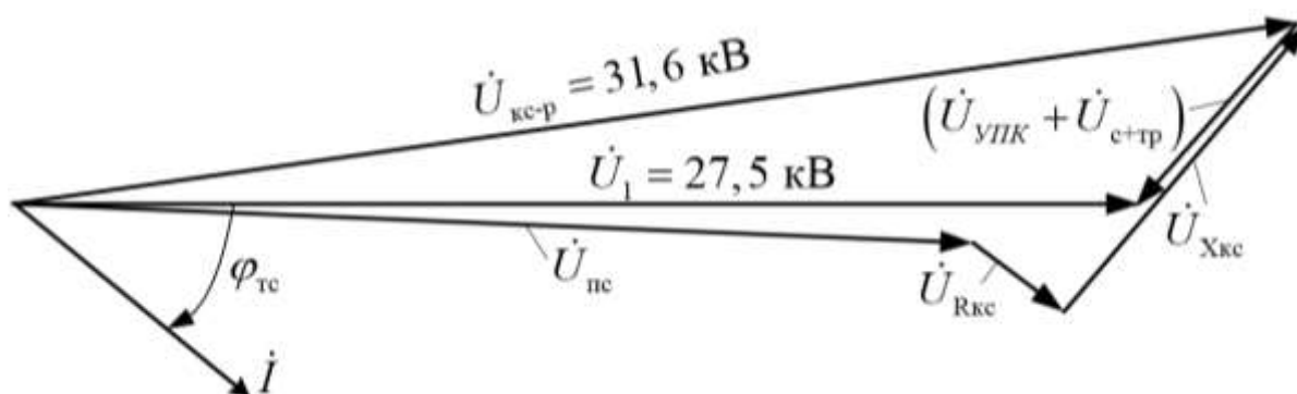
Рисунок 2 – Векторная диаграмма напряжений тяговой сети
