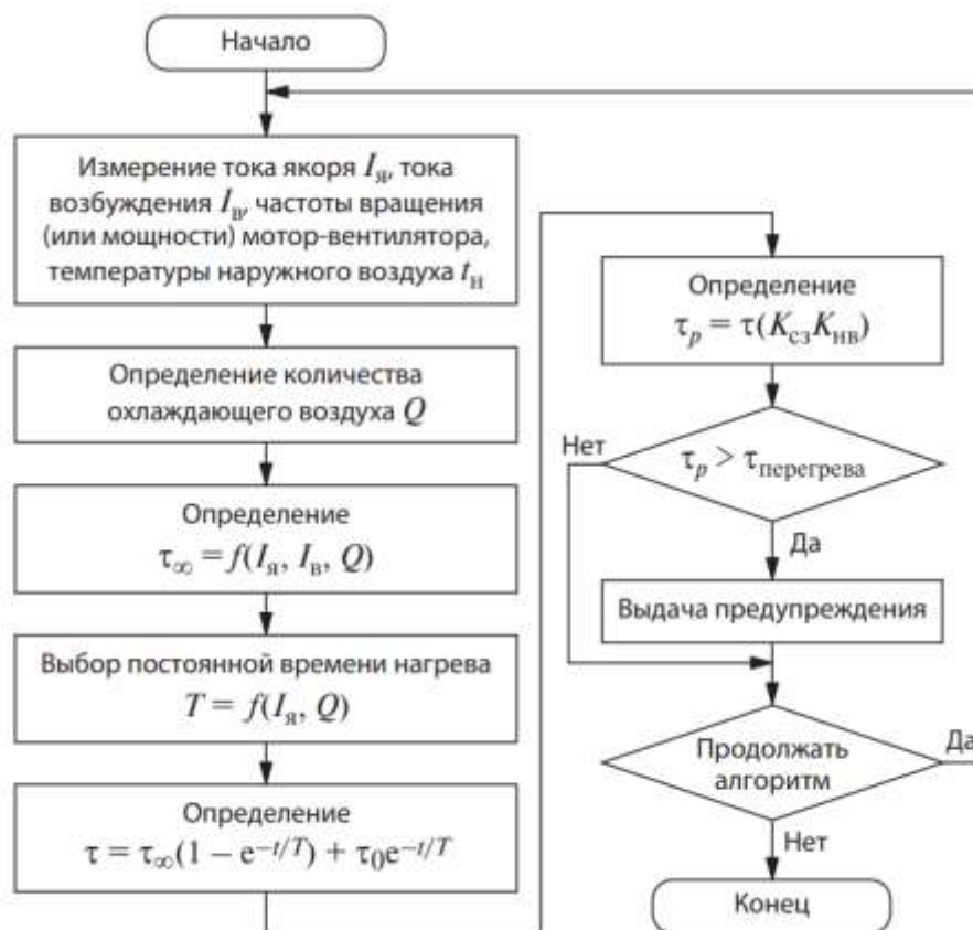
Рисунок 4 – Алгоритм определения перегрева якорной обмотки ТЭД на борту локомотива
