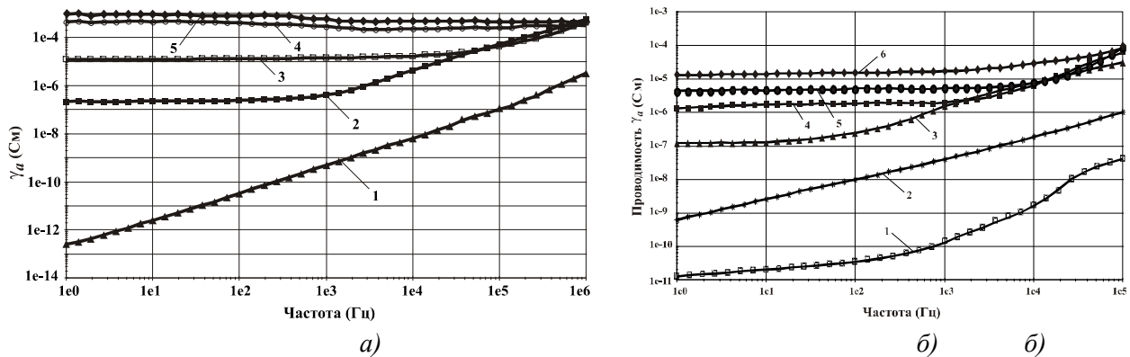
Рисунок 1 – Частотные зависимости \gamma_a : а) для ПЛА (1) и ПЛА/УНТ композиций (2-5) с различным содержанием УНТ:
