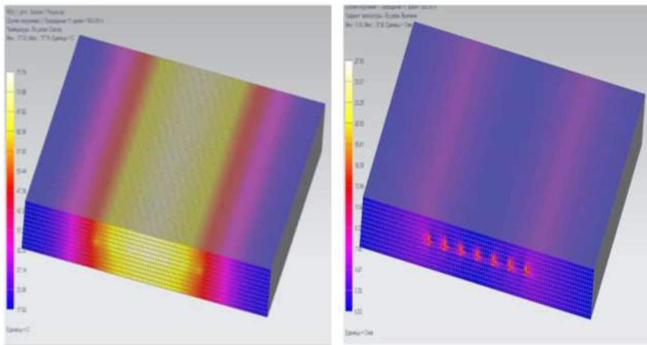
а. Поле температур в триплексе
