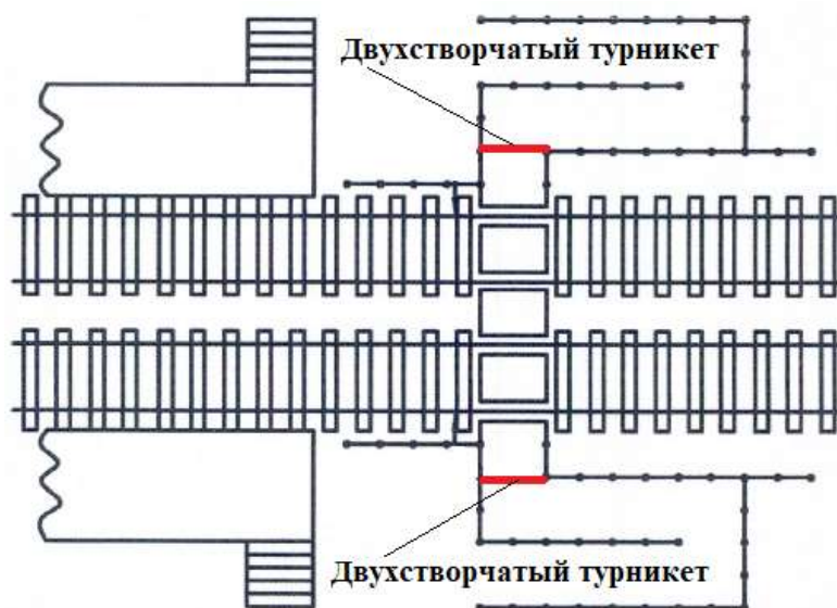
Рисунок 3 – Схема предлагаемого железнодорожного пешеходного перехода
