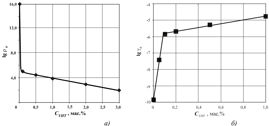
Рисунок 2 – Зависимости \rho_v = f(C_{УНТ}) для композиций ПЛА/УНТ (а)
