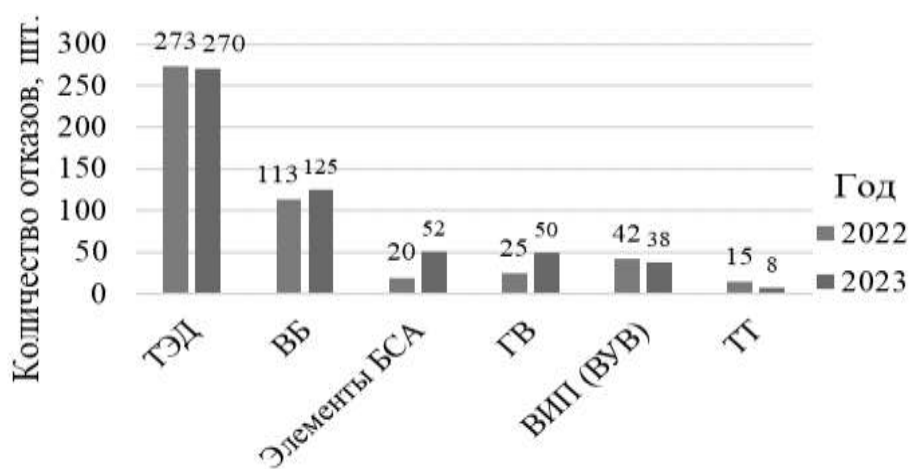
Рисунок 3 – Диаграмма распределения отказов технических средств по элементам силового оборудования локомотива 2(3)ЭС5К
