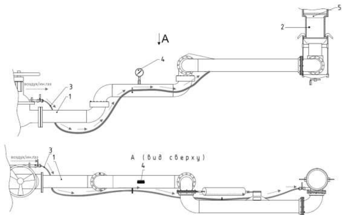
Рисунок 2 – Схема УСН с пневматической проверкой соединения
