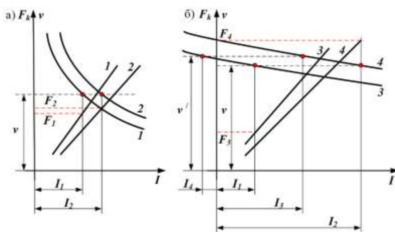
Рисунок 2 – Сравнение характеристик параллельно работающих ТЭД с последовательным и независимым возбуждением: (а) кривые 1, 2 – ТЭД последовательного возбуждения, (б) кривые 3, 4 – ТЭД независимого возбуждения
