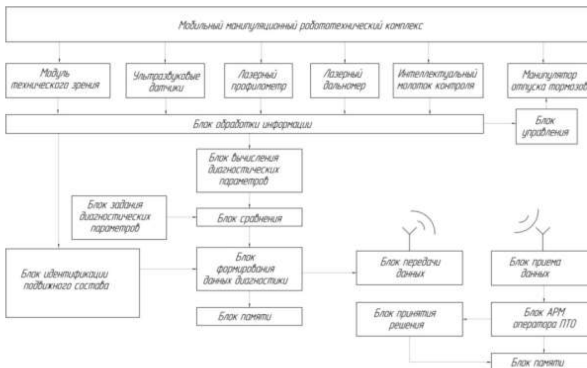
Рисунок 1 – Блок-схема аппаратно-программного устройства мобильного манипуляционного роботизированного комплекса
