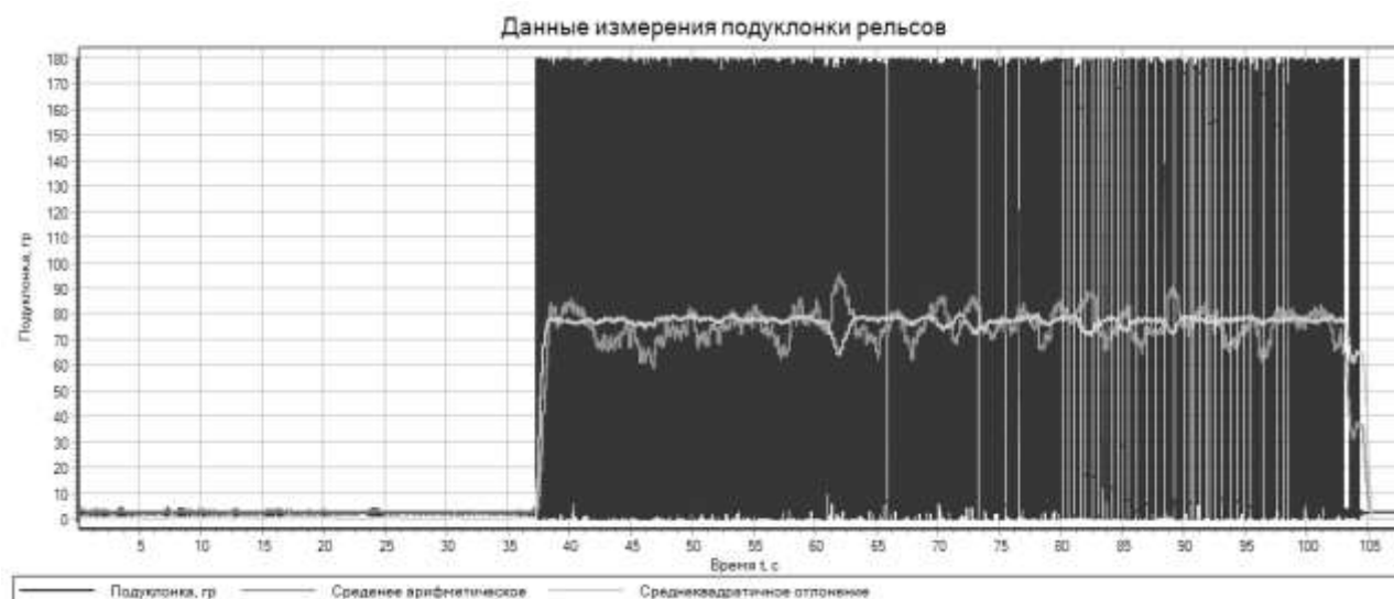
Рисунок 2 – Параметры подуклонки в динамическом режиме
