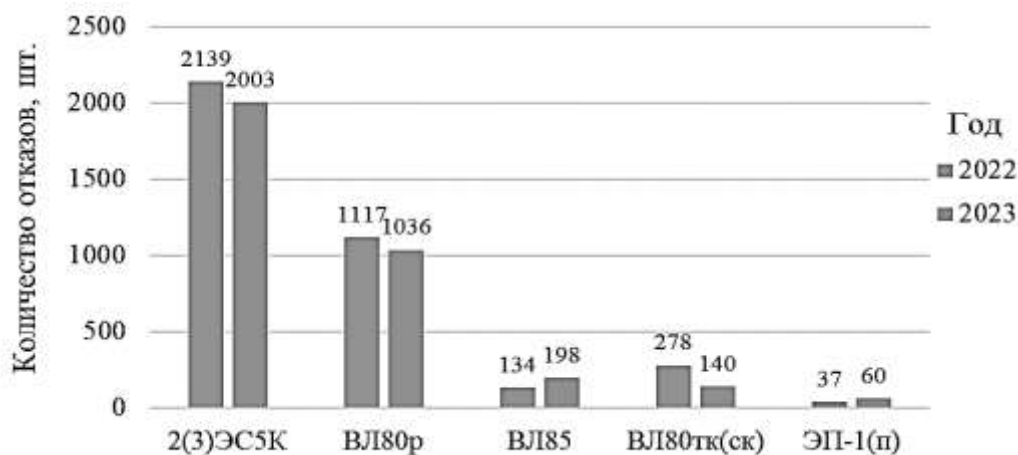
Рисунок 1 – Диаграмма отказов оборудования электровозов, эксплуатирующихся на Восточном полигоне
