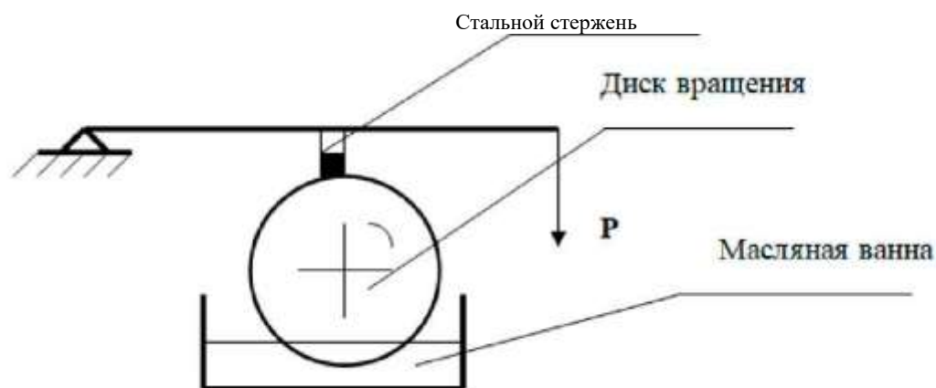
Рисунок 3 – Кинематическая схема машины для испытаний образцов масел
