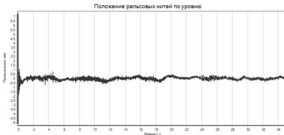
Рисунок 3 – Динамика положения рельсовых нитей по уровню под воздействием подвижного состава
