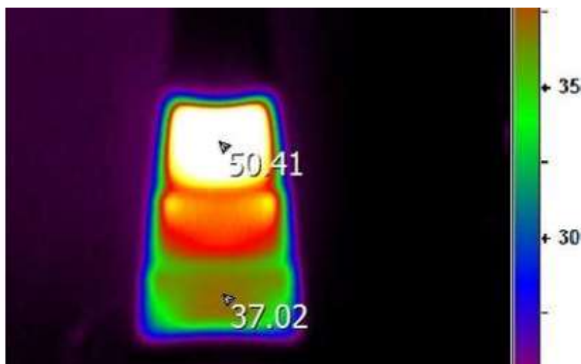
Рисунок 5 – Распределение температурного поля на поверхности стекла
