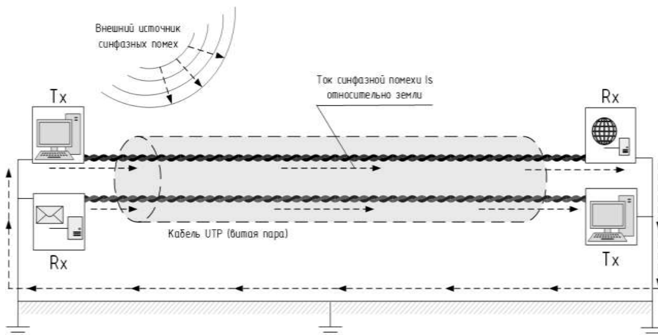
Рисунок 1 – Протекание токов синфазной помехи в несимметричной системе
