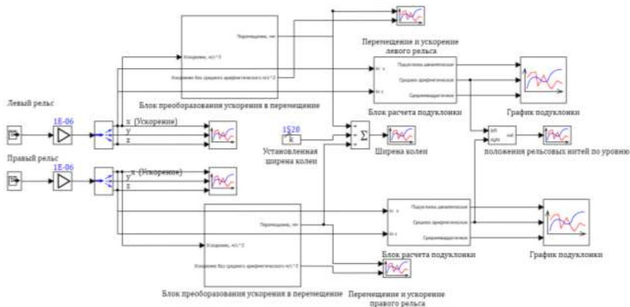
Рисунок 6 - Имитационная модель непрерывного контроля параметров рельсовой колеи в SimInTech
