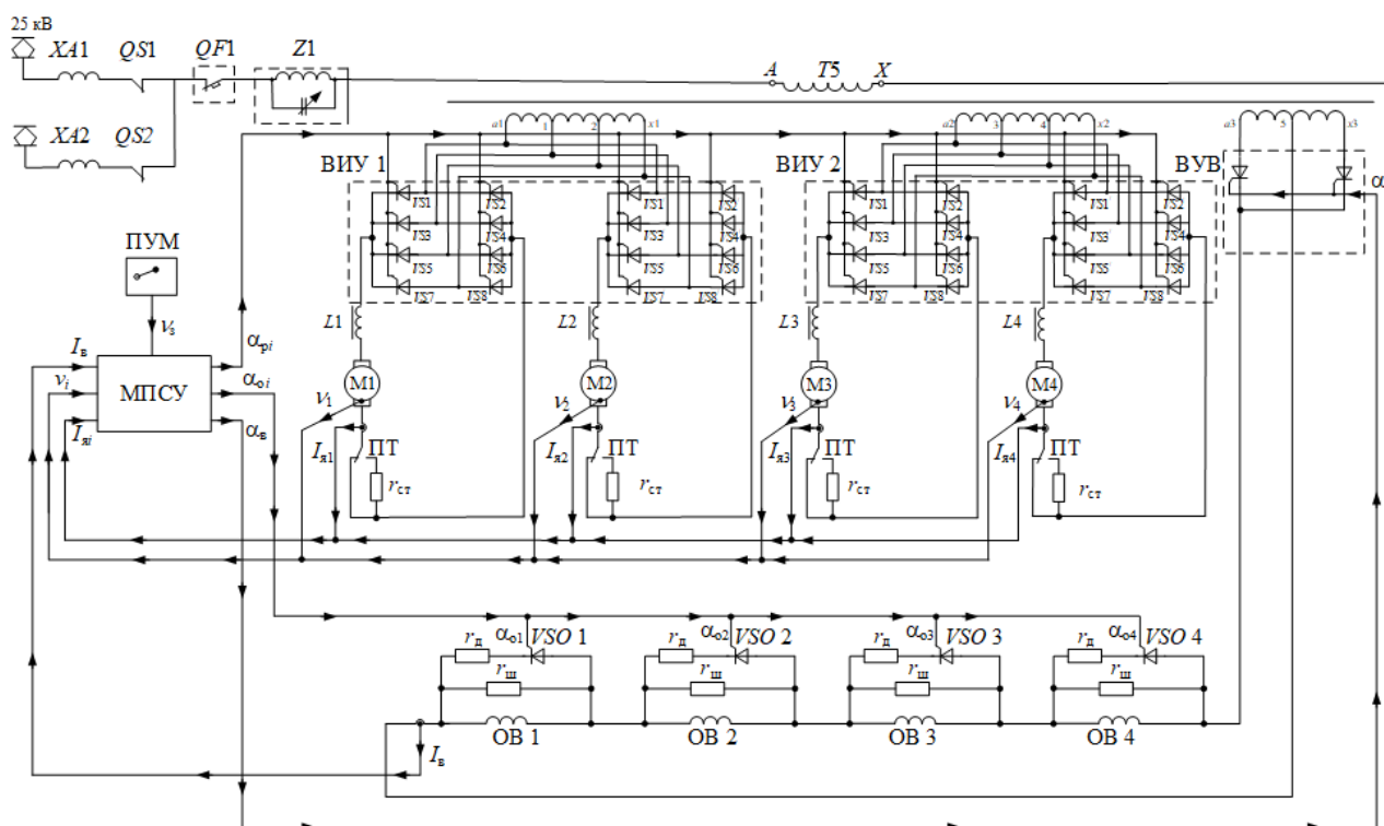
Рисунок 3 – Упрощённая схема одной секции эксплуатируемого электровоза в режиме независимого возбуждения тяговых электродвигателей
