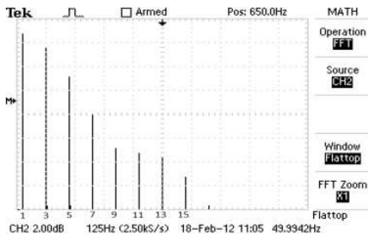
Рисунок 2 – Спектр гармоник
