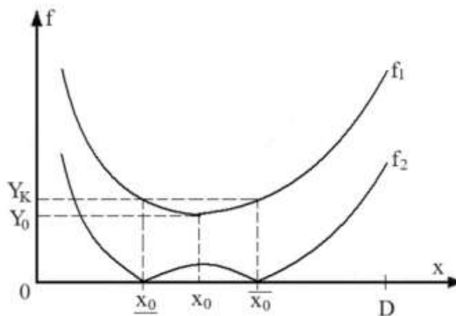
Рисунок 1 – К определению x_0 , \underline{x}_0 , \overline{x}_0 методом золотого сечения
