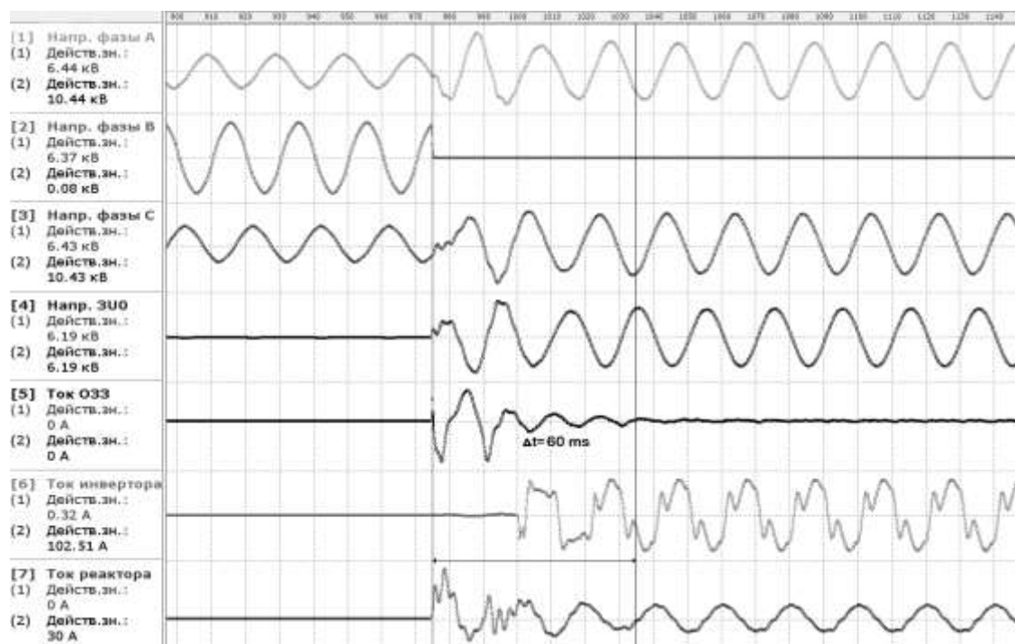
Рисунок 4 – Осциллограмма процесса компенсации тока при устойчивом ОЗЗ, полученная путем физического моделирования
