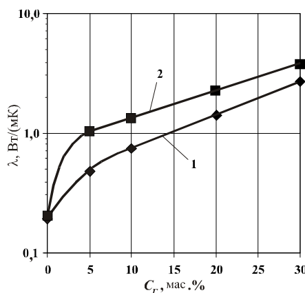
Рисунок 4 – Зависимости коэффициента теплопроводности \lambda от содержания графита для композиций ПЛА/Г: 1 – без УНТ; 2 – с 1,0 мас.% УНТ
