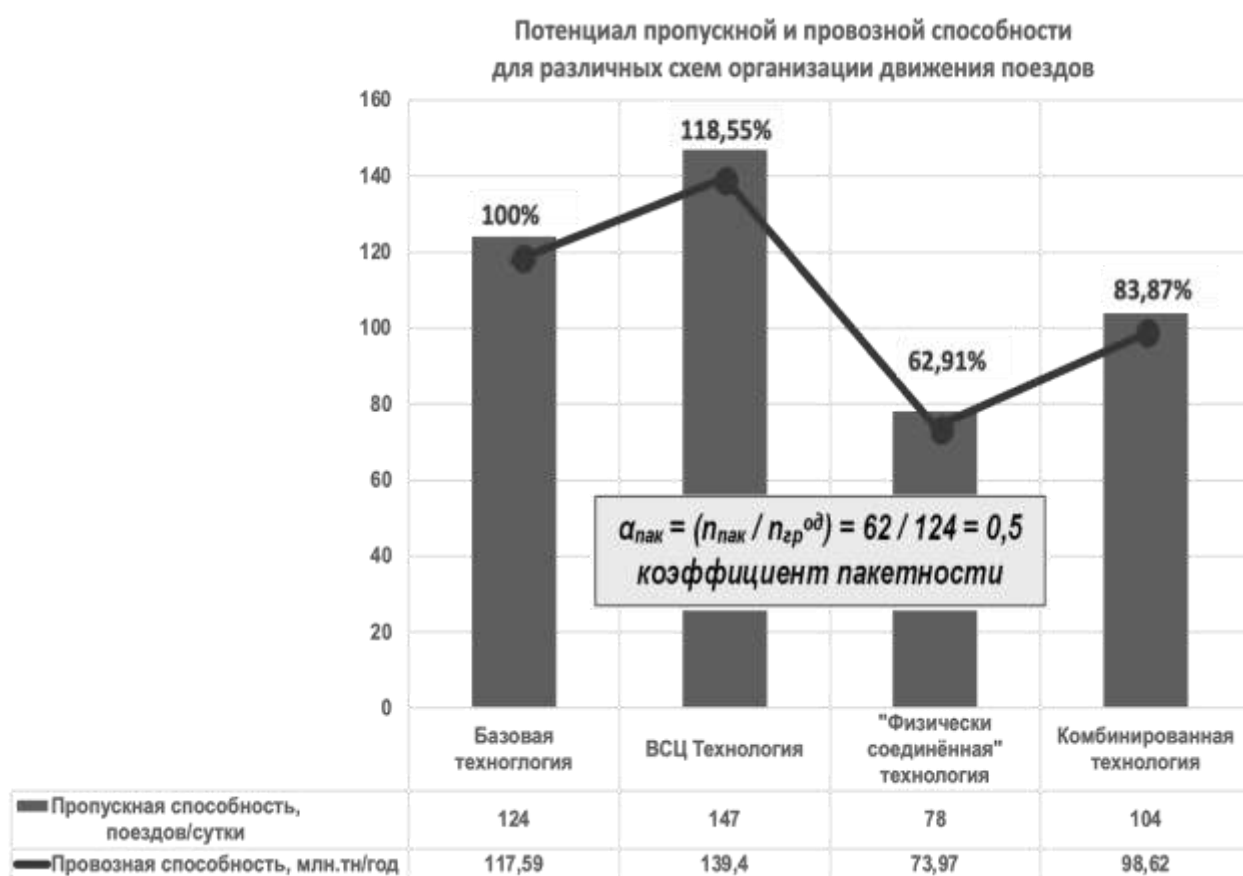
Рисунок 2 – Диаграмма соответствия пропускной и провозной способности в зависимости от используемых технологий организации движения
