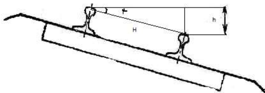
Рисунок 4 – Положение рельсовых нитей
