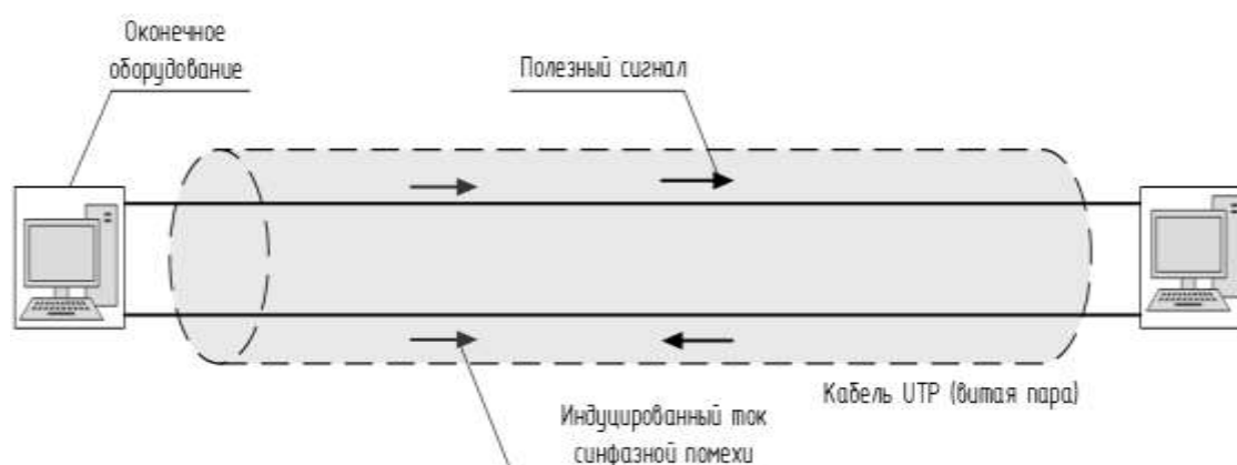
Рисунок 2 – Протекание токов синфазной помехи в симметричной линии
