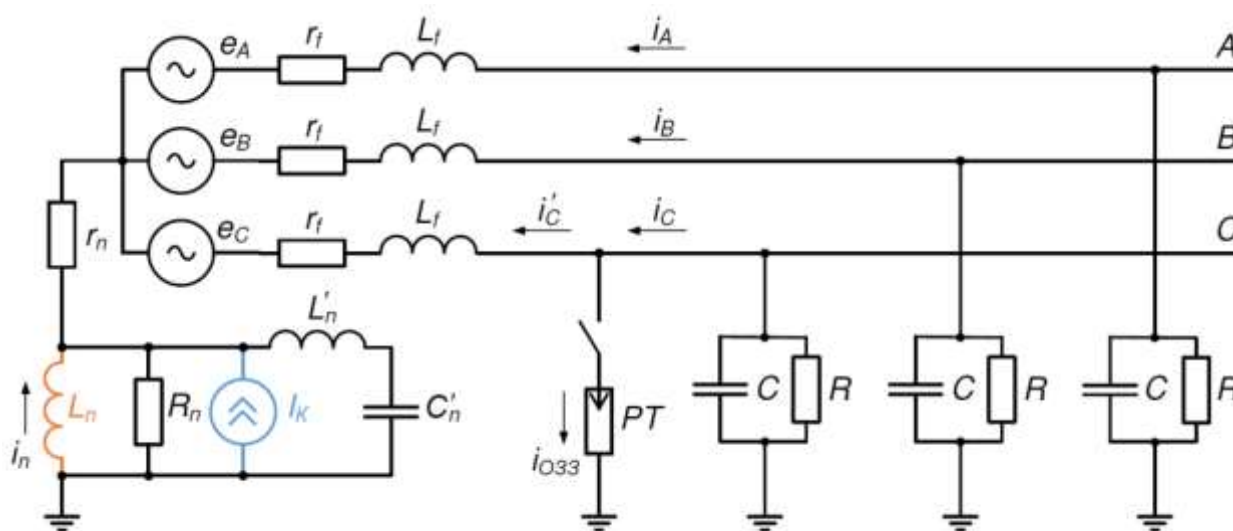
Рисунок 1 – Схема замещения сети при ОЗЗ
