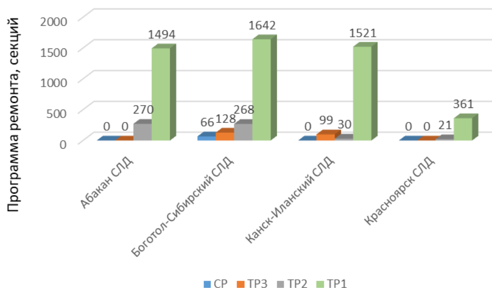
Рисунок 3 – Общее количество обслуженных секций электровозов в сервисных локомотивных депо ООО «ЛокоТех-Сервис» в границах Красноярской железной дороги за 2023 год
