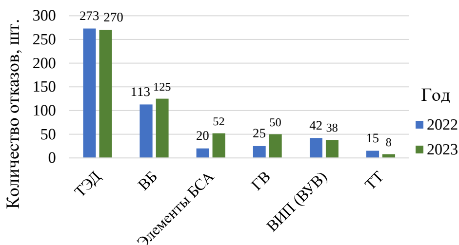
Рисунок 1– Диаграмма распределения отказов технических средств по элементам силового оборудования локомотива 2(3)ЭС5К приписки Красноярской дирекции тяги
