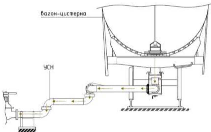
Рисунок 1 – Схема слива нефтепродуктов из железнодорожных цистерн
