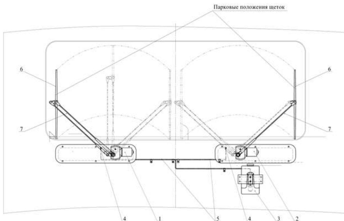
Рисунок 1 – Система для очистки лобовых стекол
