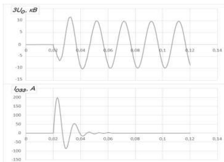
Рисунок 3 – Осциллограмма процесса компенсации тока при устойчивом ОЗЗ, полученная путем математического моделирования
