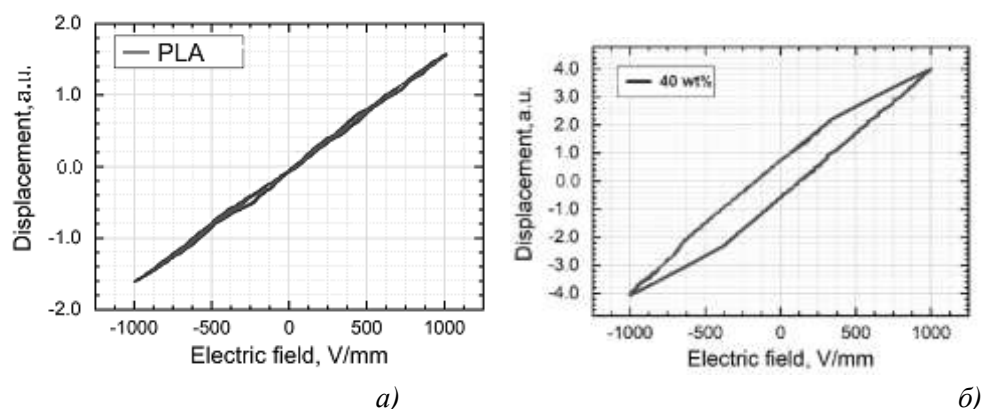
Рисунок 7 – Петли диэлектрического гистерезиса: а) ПЛА; б) ПЛА+40 мас.%ТБ
