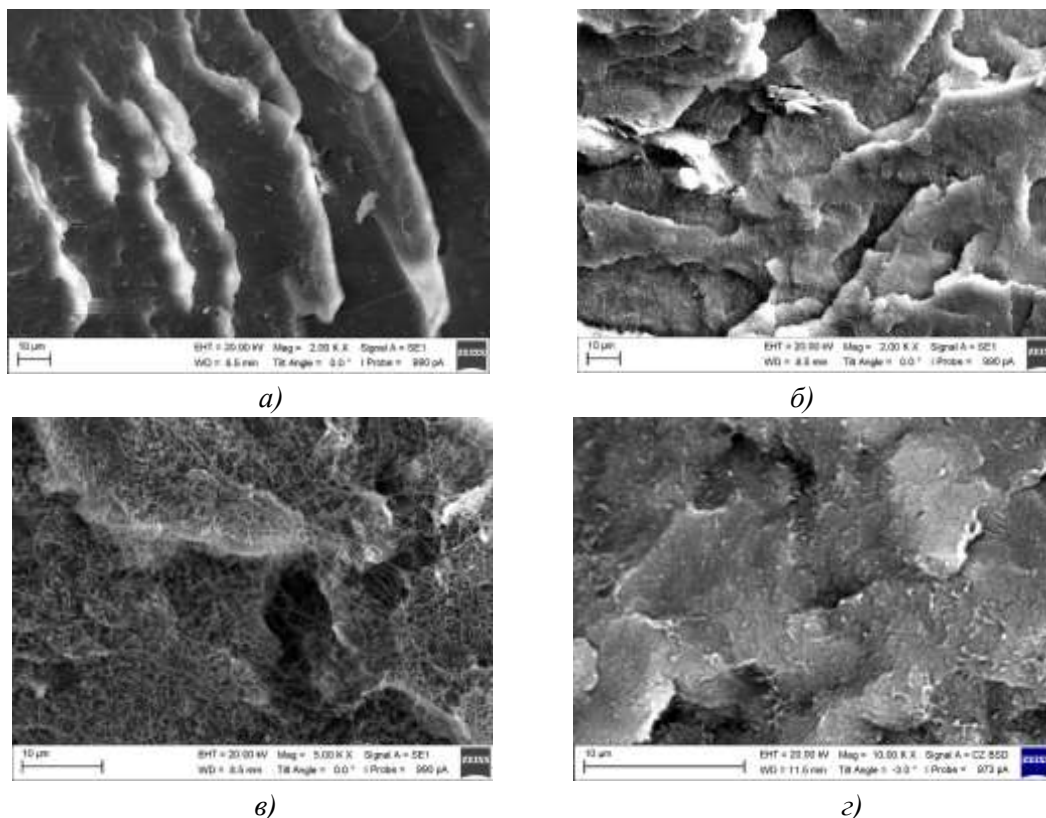
Рисунок 3 – СЭМ микрофотографии для композиций ПЛА/УНТ (а-г):
