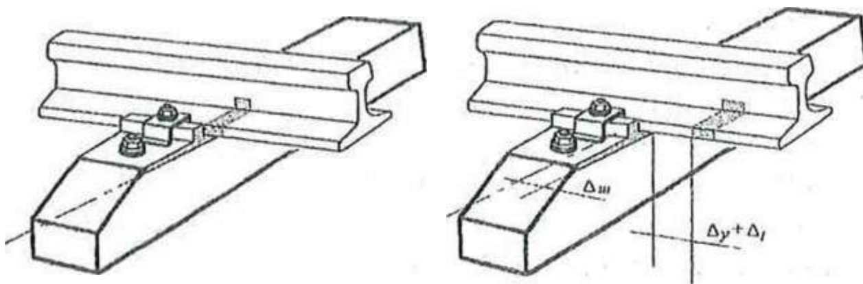
Рисунок 1 – Измерение перемещений рисок на маячной шпале
