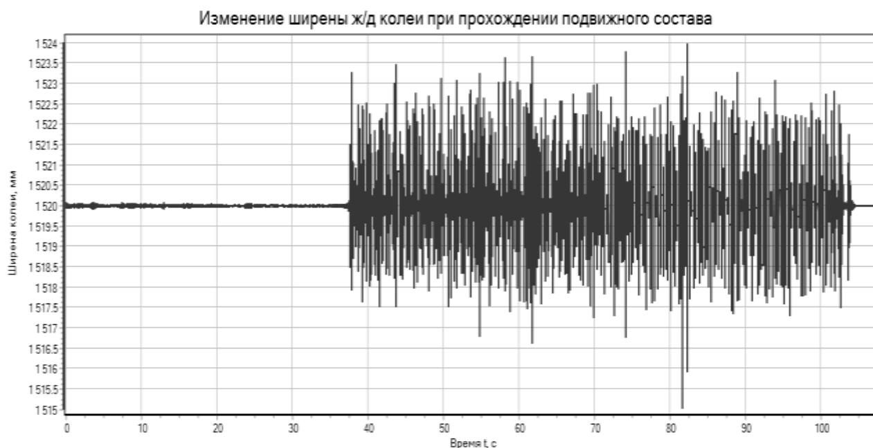
Рисунок 5 - Динамические изменения ширины железнодорожной рельсовой колеи под воздействием подвижного состава
