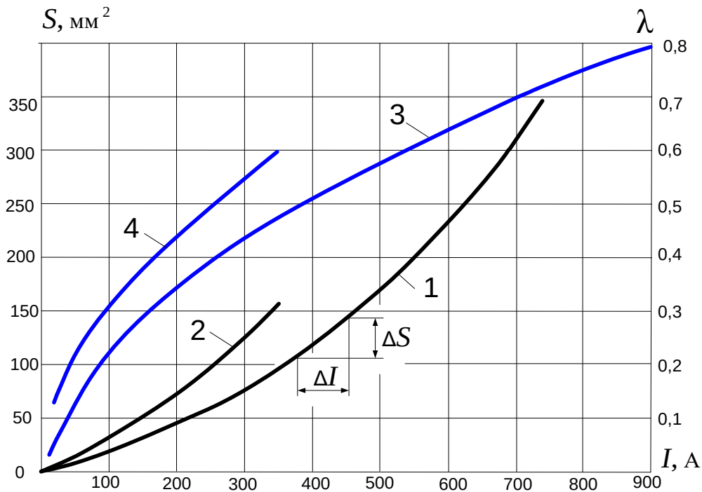
Рисунок 1 – Зависимость сечения обмотки (1, 2) и коэффициентов \lambda (3, 4) от тока: 1, 3 – медный провод; 2, 4 – алюминиевый провод
