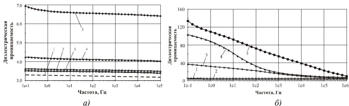
Рисунок 6 – Частотные зависимости \varepsilon' для ПЛА и композиций ПЛА/ТБ (а): 1 – ПЛА; 2 – 5 % ТБ; 3 – 10 % ТБ; 4 – 20% ТБ; 5 – 40% ТБ; и ПЛА/ТБ/УНТ (б): 1 – ПЛА; 2 – 5 % ТБ; 3 – 10 % ТБ; 4 – 20% ТБ; 5 – 40% ТБ
