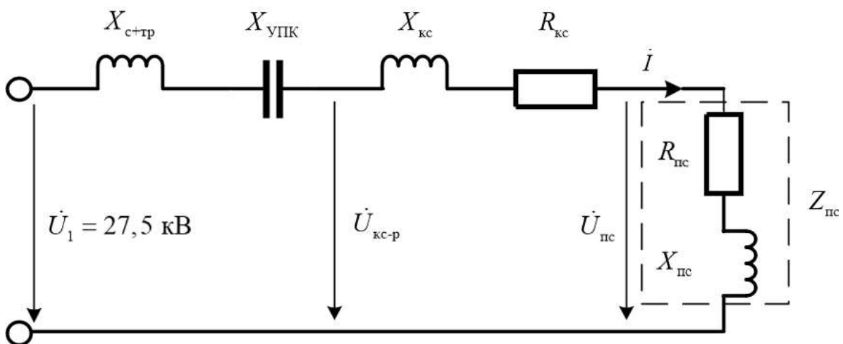
Рисунок 1 – Схема замещения тяговой сети
