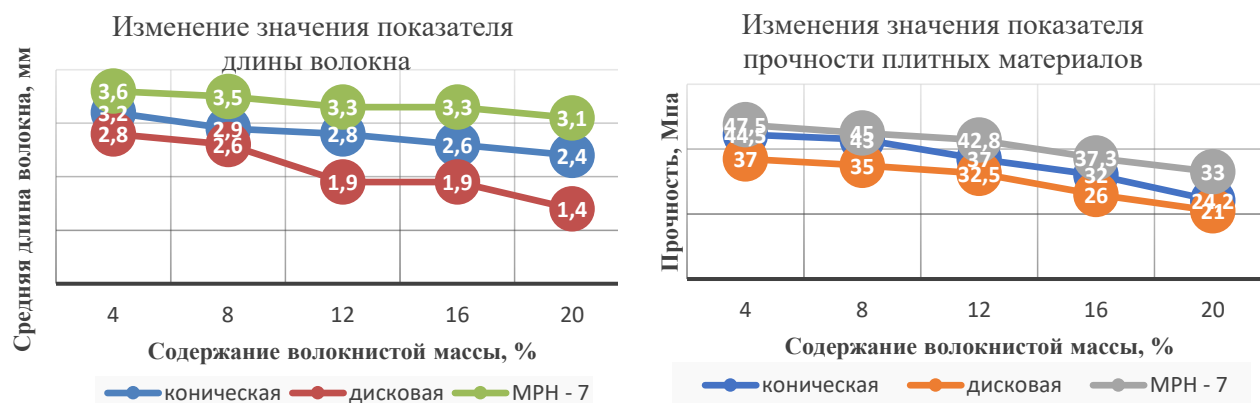
Рисунок 3 - Показатели значений оцениваемых факторов от содержания вторичной массы в пресс-композиции при различных способах обработки волокна
