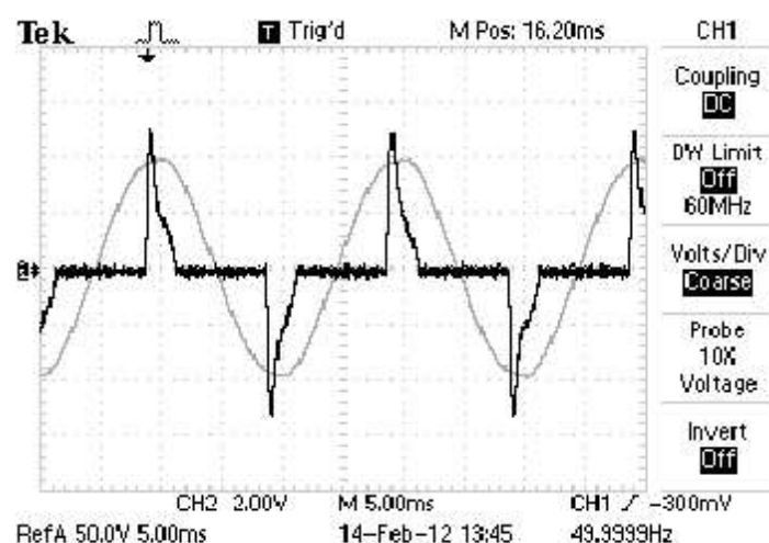
Рисунок 1 – Гармонические составляющие
