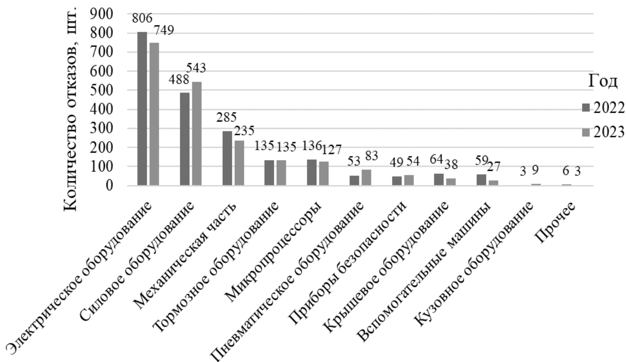
Рисунок 2 – Диаграмма отказов технических средств по видам оборудования локомотива 2(3)ЭС5К
